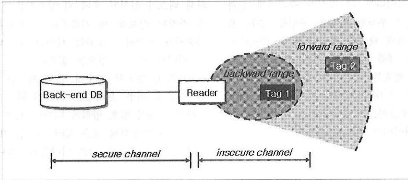
그림 1. RFID 시스템
