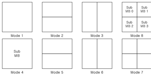
그림 2. 움직임 추정에 사용되는 다양한 크기의 매크로블록 모드 Fig. 2. The macroblock mode with the VBS (Variable Block Size) for the motion estimation
