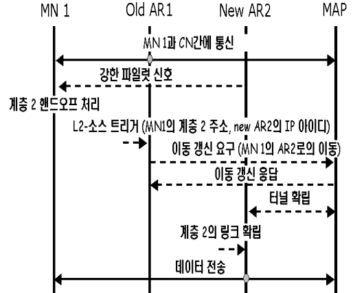
그림 5. 그룹 상태에서의 메시지 흐름도
