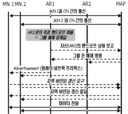
그림 6. 그룹 해제 상태에서의 메시지 흐름도
