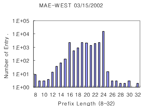
그림 1. 프리픽스 분포
