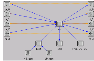
(b) 노드 모델
