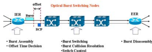
그림 1. 광 버스트 스위칭 망
