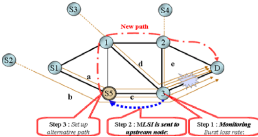
그림 3. 망 상태 모니터링을 통한 MLSI 메시지 전송기법
