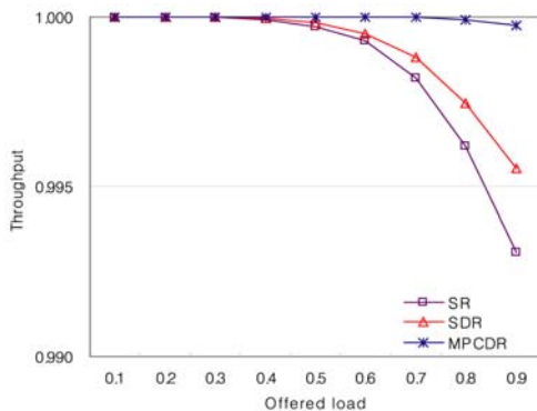
그림 12. HB 처리율 (HB(30%):LB(70%))
