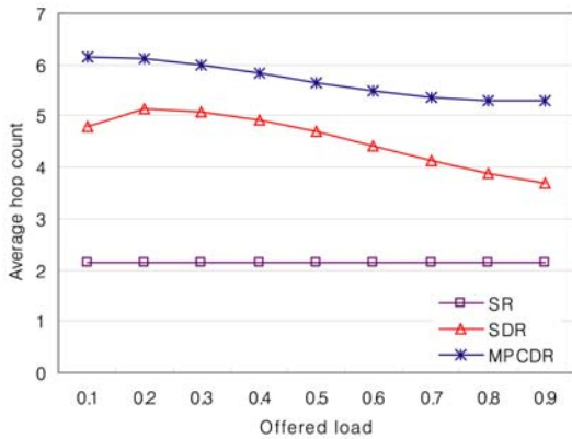
그림 14. 평균 홉 수
