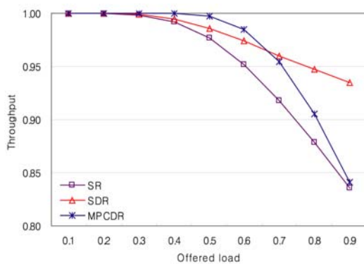
그림 13. HB 처리율 (HB(70%):LB(30%))
