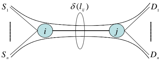
그림 7. link-degree 개념
