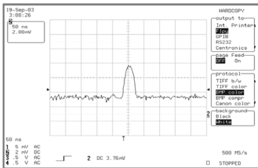
(a) 파장 변환된 데이터 신호
