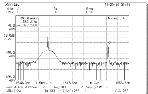
(b) 동시 입사되는 광펄스들의 스펙트럼
