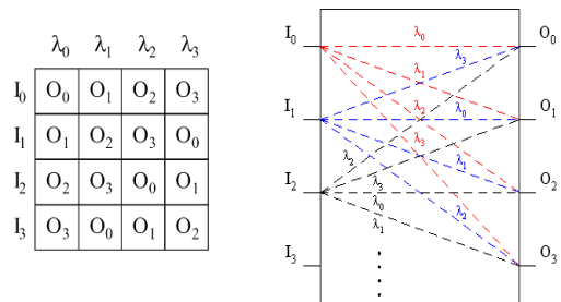
그림 3. AWG의 라우팅 규칙
