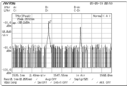
(b) 최종 출력 스펙트럼
