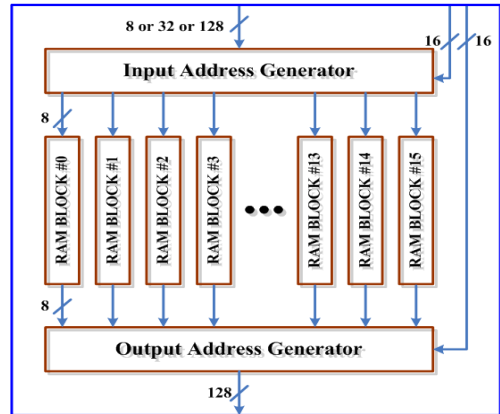
그림 4. 인터 메모리의 구조
