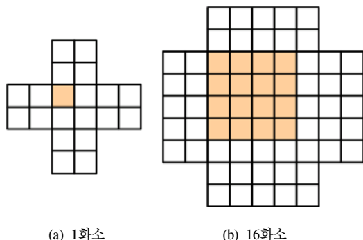
(a) 1화소 (b) 16화소 그림 7. 6단 FIR 필터계산을 위한 데이터양
