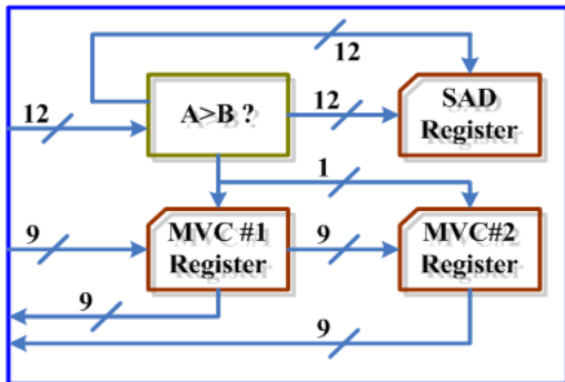
그림 12. 레벨 2를 위한 비교기 구조
