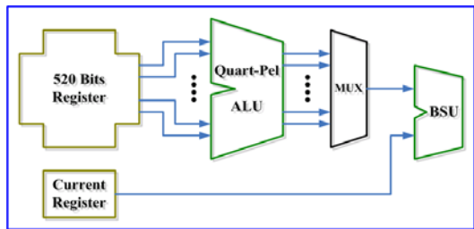
그림 10. 1/4화소 단위 고속 블록 계산 흐름도
