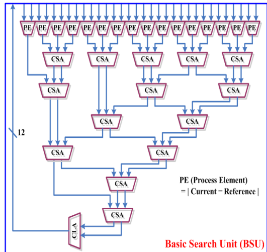
그림 6. BSU의 구조
