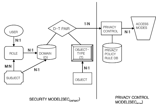
그림 2. 제안된 모델
