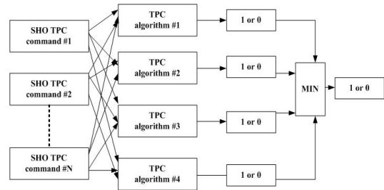
그림 2. 다양한 TPC 알고리즘의 병렬 사용
