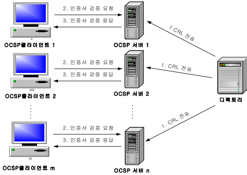
그림 6. 분산 OCSP서버 CRL정보 송수신 과정
