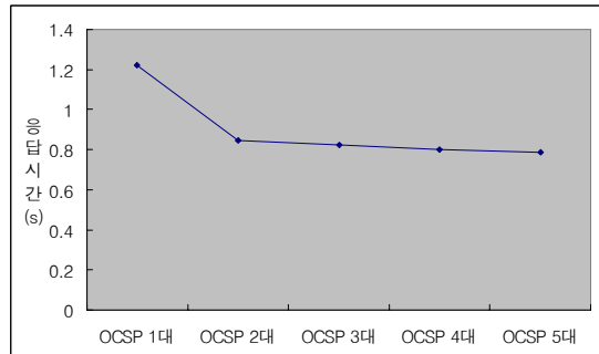
그림 10. 인증서 상태 검증 서비스 요청에 대한 응답시간
