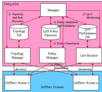
그림 2. PMQoSs의 개념적 관리 구조 Fig 2. Conceptual QoS management architecture of PMQoSs
