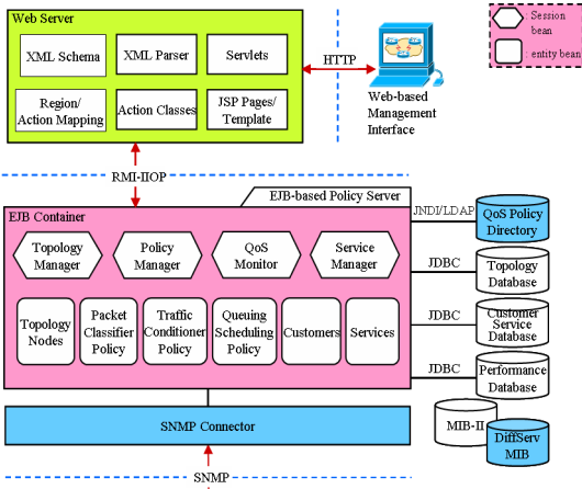
그림 1. PMQoSs의 QoS 관리 구현 구조 Fig 1. Implemental QoS management architecture of PMQoSs
