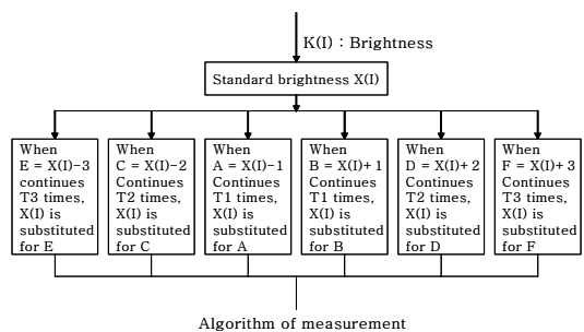
그림 4. 기준 휘도치의 자동조정기법의 흐름도
