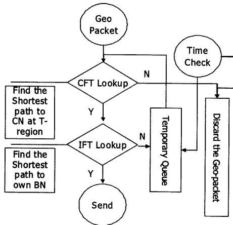
그림 4. 지오패킷 전달 과정도
