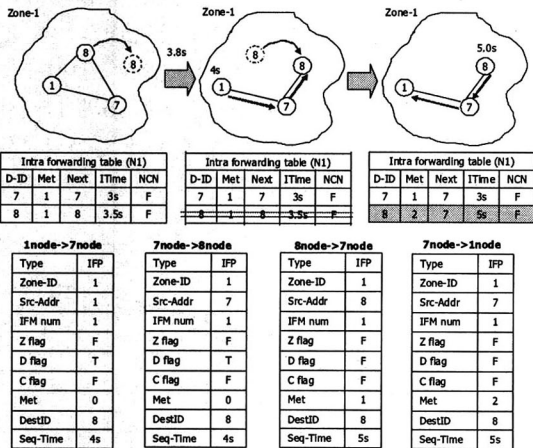
그림 7. 동일 CN내에서의 경로 재설정 설명도
