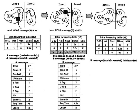
그림 8. 이웃 CN 추가 과정 설명도
