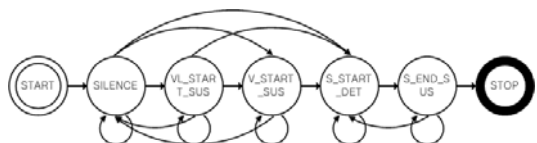
그림 1. 입력음성신호에서 발화 검출을 위한 상태도
