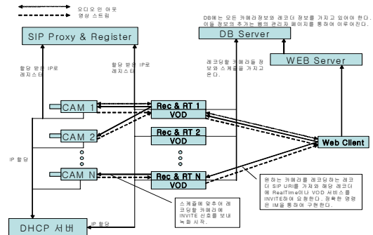
그림 2. 전체 시스템 구성도
