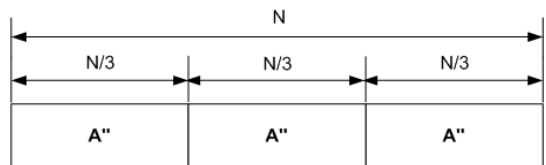
그림 1. 시간 영역에서 3번 반복되는 프리앰블 구조 (Preamble).
