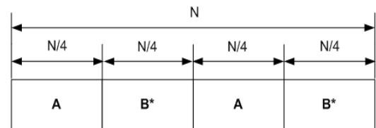
그림 4. 시간 영역에서의 제안된 프리앰블 구조 (Preamble p ).
