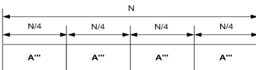
그림 3. 시간 영역에서 4번 반복되는 프리앰블 구조 (Preamble 4 ).
