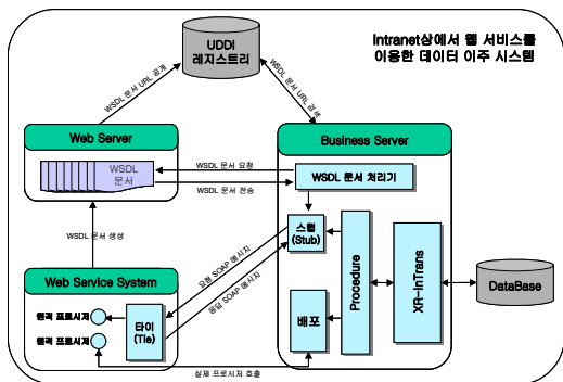
그림 1. 웹 서비스를 이용한 데이터 이주 시스템 전체 구성도
