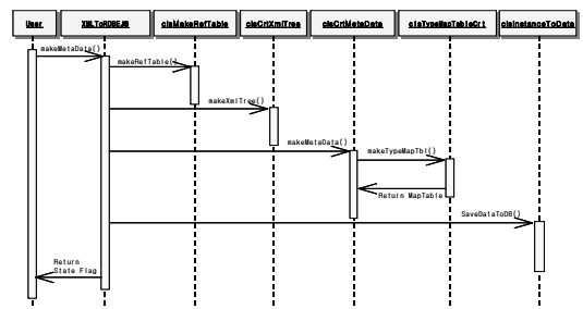
그림 11. XMLToRDB 순차 다이어그램
