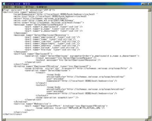
그림 16. 웹 서비스에서 작성된 WSDL 문서
