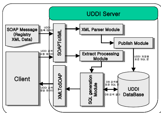
그림 7. UDDI Server System 구조
