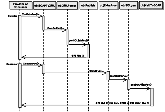
그림 12. UDDI 레지스트리 등록 및 검색 순차 다이어그램
