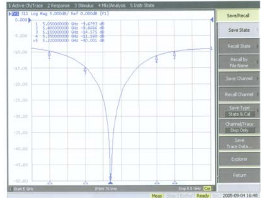
그림 7. Measured return loss
