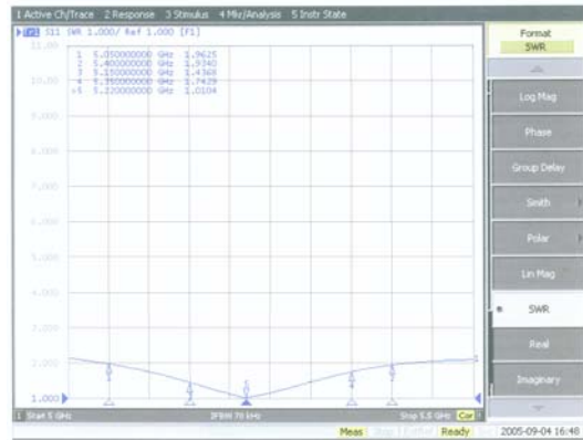
그림 8. Measured VSWR
