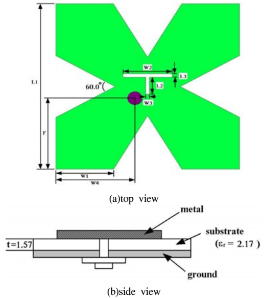
그림 1. Antenna configuration
