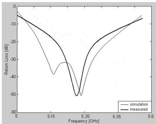
그림 5. Compare the simulation with measured result
