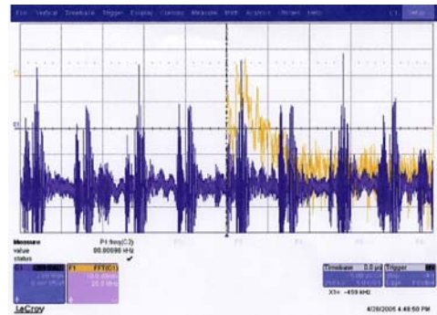
그림 8. R-L-C 필터를 사용한 경우의 캐소드 리플 파형
