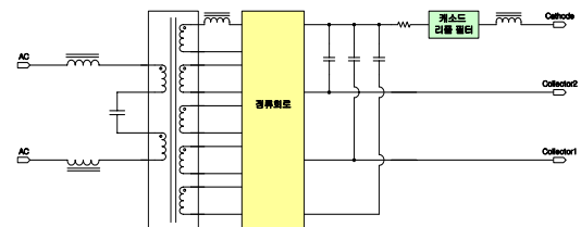
그림 3. 고압전원모듈 구성도
