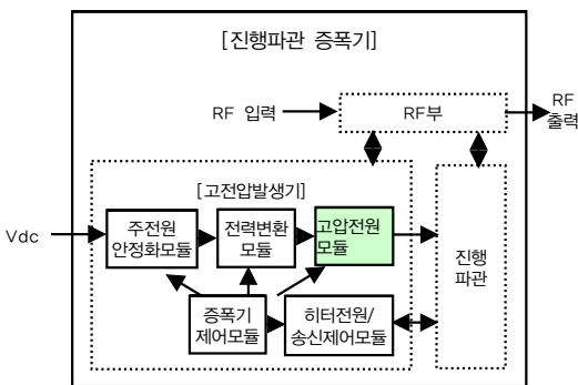
(b) 구성도
