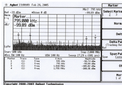
그림 5. 필터가 없는 경우의 잔류 AM
