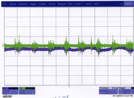
그림 16. 개선 후의 +15V 리플 잡음.
