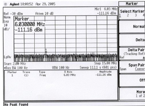
그림 12. 잔류 AM 측정 결과(2MHz~15MHz).
