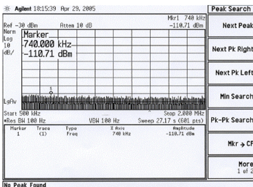
그림 11. 잔류 AM 측정 결과(500KHz ~ 2MHz)
