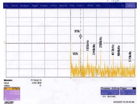
그림 9. 캐소드 리플파형의 FFT 스펙트럼
