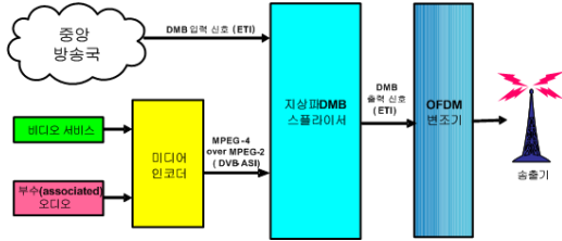
그림 4. 지상파DMB 스플라이싱 시스템 블록도
