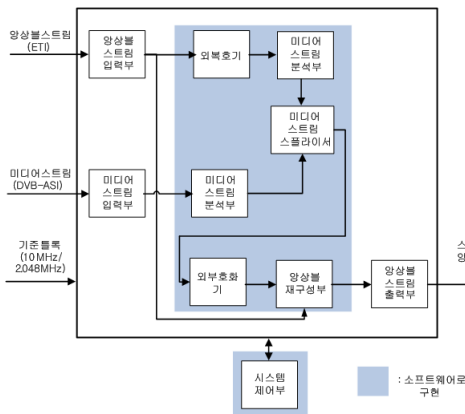
그림 5. 지상파DMB 스플라이서 구조
