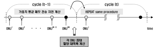
그림 2. 적응적 Limited 방식의 개념도
