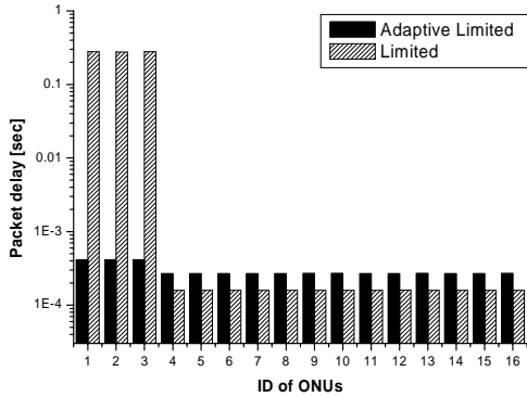
그림 9. 불균형적인 트래픽 환경에서의 각 ONU별 평균 패킷 전송 지연
