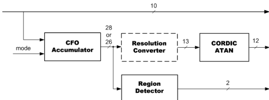
그림 2. 반송파 주파수 오프셋 추정부의 구현 블록도
