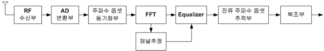
그림 1. IEEE 802.11a의 수신부 블록도
