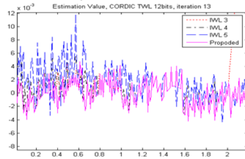
그림 7. Compact CORDIC 전처리부 추정 성능
