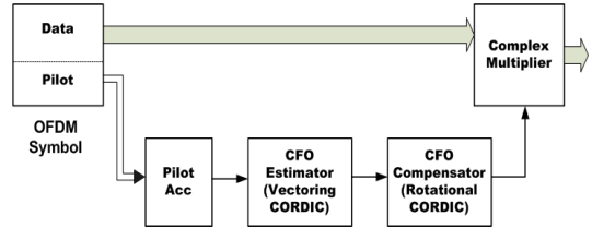
그림 3. 잔류 주파수 오프셋 추정 및 보상부 블록도
