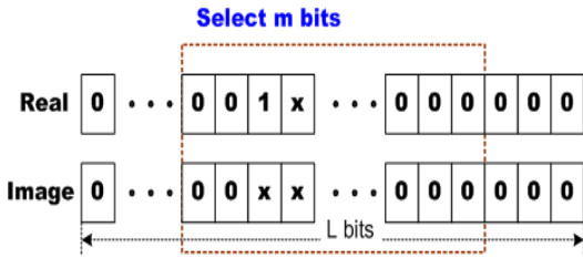
그림 4. Compact CORDIC 전처리부
