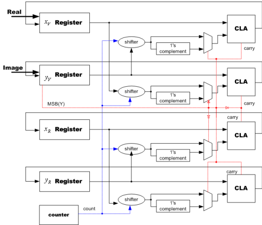
그림 6. Compact CORDIC processor 블록도
