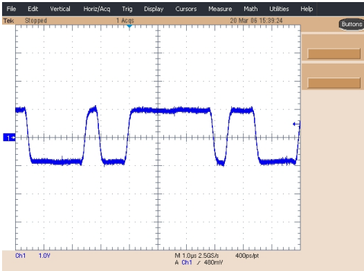
그림 15. 교정된 pre-modulation 필터를 적용한 최종 2Mbps 비트스트림 파형 Figure 15. Calibrated filtered_out waveform when bit rate is 2Mbps
