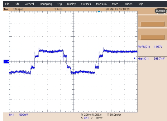
그림 11. FIR 필터 및 DAC 시스템 출력파형 Figure 11. Output waveform of FIR filter and DAC system
