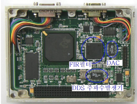
그림 16. 구현된 RF 인터페이스 PCB 보드 Figure 16. Implemented RF interface PCB 1
