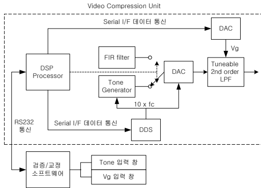
그림 7. 아날로그 변환부의 검증 및 교정을 위한 구성도 Figure 7. Block diagram for the verification and calibration of analog conversion part
