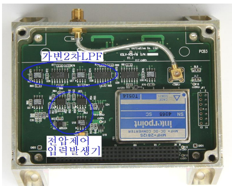
그림 17. 구현된 RF 인터페이스 PCB 보드2 Figure 17. Implemented RF interface PCB 2
