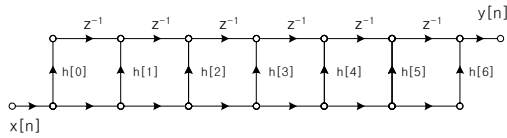
그림 3. 적용된 FIR 필터 구조 Figure 3. Adopted FIR filter structure
