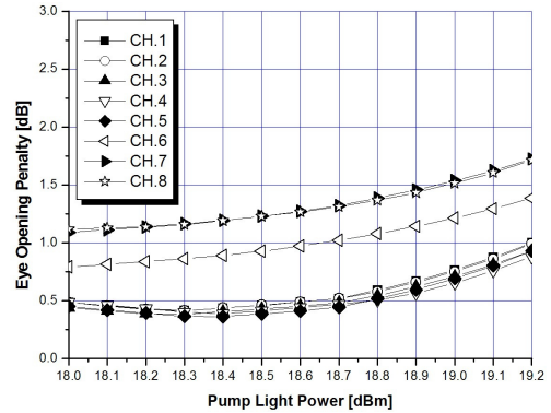
(b) l=100 km ; D=1.6 ps/nm/km ; RZ
