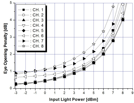
(d) D=1.6 ps/nm/km ; P_p=17.95 dBm
