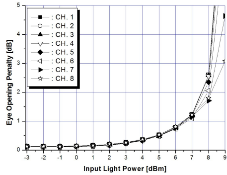
(f) D=0.4 ps/nm/km ; P_p=18.54 dBm
