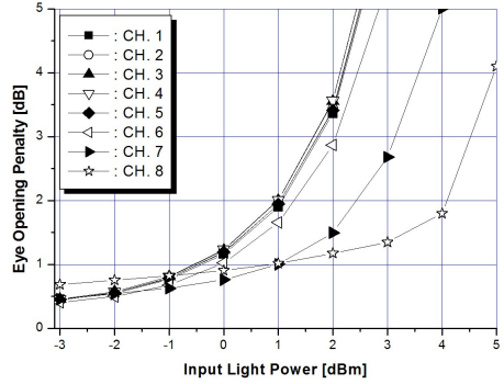
(d) D=1.6 ps/nm/km ; P_p=18.63 dBm
