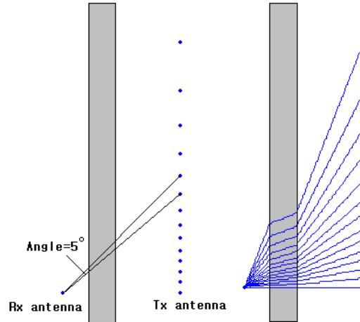
그림 2. 측정계획 (왼쪽)과 모의실험에 의해 찾아진 전파경로 (오른쪽)
