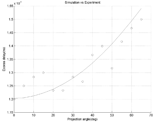
그림 3. 직선경로 신호의 도착시간의 측정치와 모의실험 결과 비교
