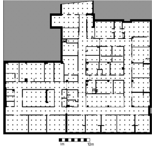
그림 4. 통계적모델링을 위해 사용된 Jesus Hospital의 도면. 그림에 나타난 점들은 가상의 송수신기의 위치를 나타낸다.
