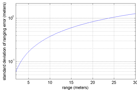
그림 6. 거리추정 오차의 편차의 CRLB.
