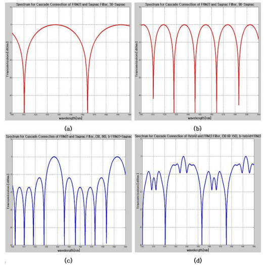
그림 4. 기존의 Sagnac 필터와 제안된 필터들간의 통과 스펙트럼 비교 (a) Sagnac 필터만을 사용했을 경우(거리차 = 30\mu\text{m} 일때) (b) Sagnac 필터만을 사용했을 경우(거리차 = 90\mu\text{m} 일때), (c) FRMZI + Sagnac 필터의 경우( \Delta L1=30\mu\text{m} , \Delta L2=90\mu\text{m} ), (d) 하이브리드 필터 + FRMZI의 경우( \Delta L1=30\mu\text{m} , \Delta L2=60\mu\text{m} , \Delta L3=150\mu\text{m} )
