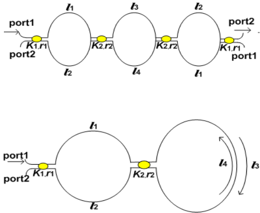
그림 3. FRMZI를 일반화한 후에 전개한 다이어그램
