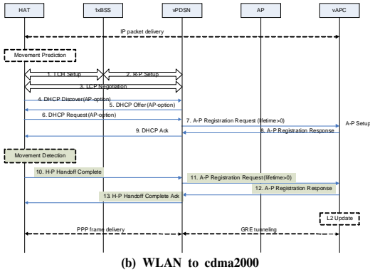
그림 3. 제안하는 핸드오프 절차
