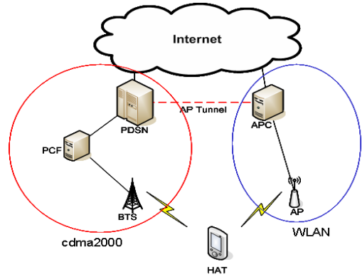
그림 2. 제안하는 연동망 구조
