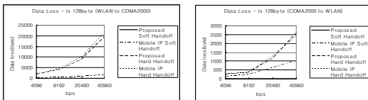
그림 8. 핸드오프시의 패킷 손실
