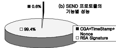
그림 8. SEND 프로토콜의 성능 Fig. 8. Performance of SEND protocol
