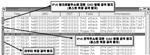
그림 7. IP 자동구성 방해공격의 탐지 Fig. 7. Detection of attacks against IP auto-configuration
