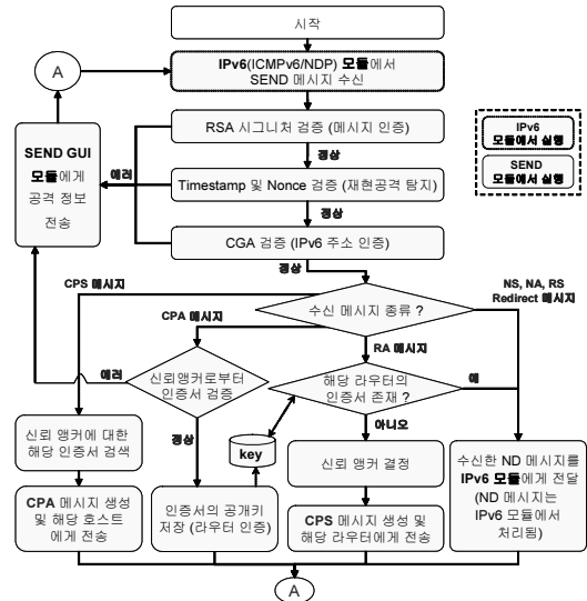
그림 4. 수신한 SEND 메시지의 처리 알고리즘 Fig. 4. Algorithm for SEND message processing in a receiver system
