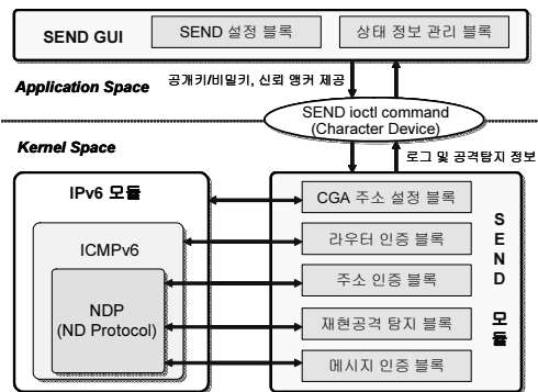
그림 2. SEND 프로토콜을 위한 IPv6 시스템의 구조 Fig. 2. Architecture of IPv6 system for SEND protocol
