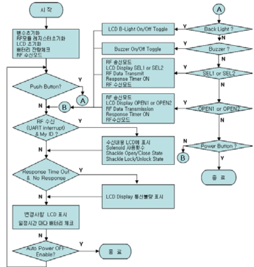
그림 6. 원격 제어기 프로그램 순서도
