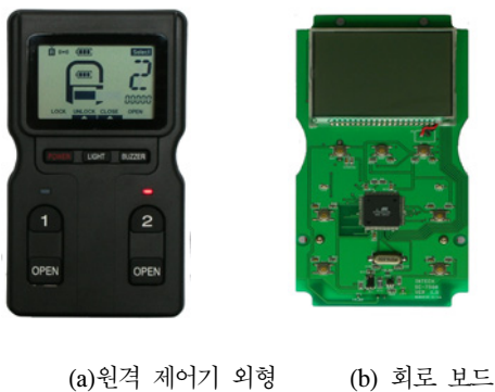
그림 9. 제작된 원격 제어기 회로 보드와 외형 모습
