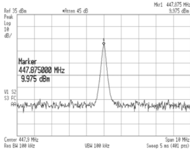
(a) 출력 파워 및 주파수
