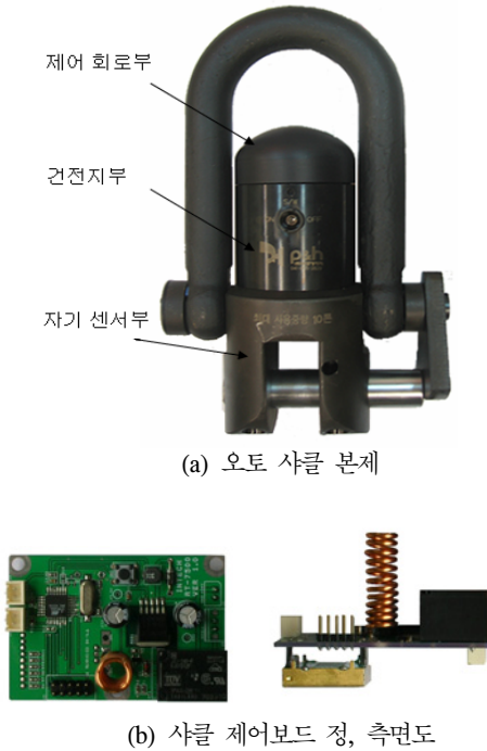
그림 8. 제작된 샤클과 내장된 제어 보드 모습
