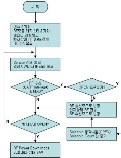
그림 5. 샤클내 제어부 프로그램 순서도
