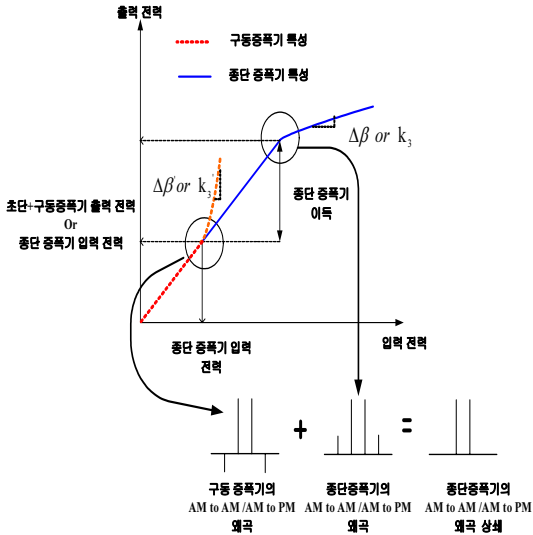
그림 3. 전력 증폭기의 왜곡 상쇄 원리
