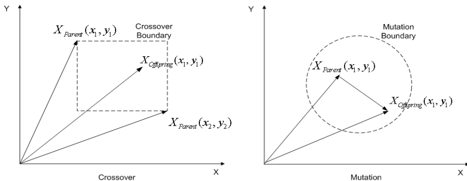
그림 2. 유전 알고리즘의 교차와 돌연변이 연산과정
