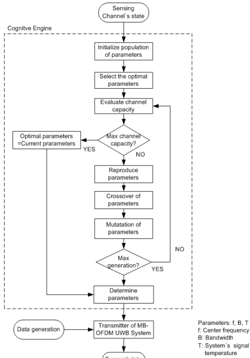
그림 4. 유전 알고리즘 연산 순서도
