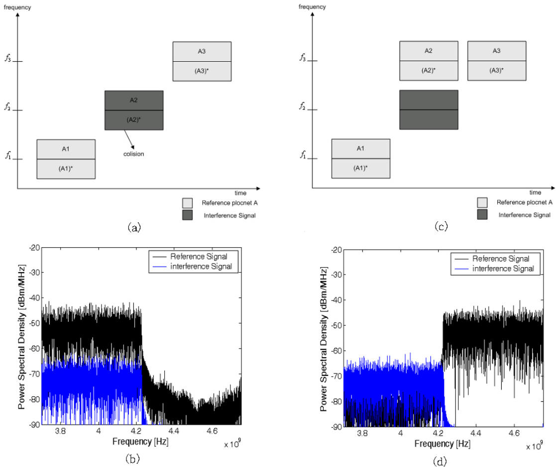
그림 6. UWB 신호간의 간섭상황 및 간섭회피
