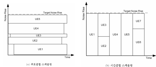
그림 1. 부호분할 스케줄링과 시간분할 스케줄링의 자원 할당방식
