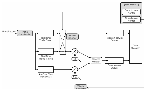
그림 2. 실시간 트래픽의 QoS 보장을 위한 하이브리드 스케줄러의 구조
