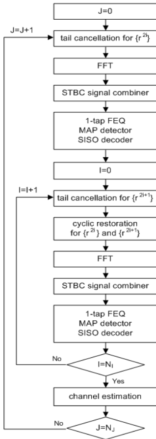
그림 4. 채널 추정을 포함한 STBC OFDM 잔재 ISI 제거 기법 ( N_j = 잔재 ISI 제거 반복 횟수, N_j = 채널 추정 반복 횟수)
