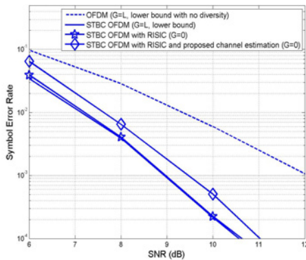
그림 9. CH_2 채널에 대한 STBC OFDM 시스템의 심볼 에러율 성능
