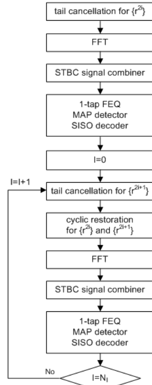
그림 2. STBC OFDM을 위한 잔재 ISI 제거 기법 ( N_T = 반복 횟수)
