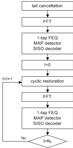
그림 1. 잔재 ISI 제거 기법 ( N_i = 반복 횟수)
