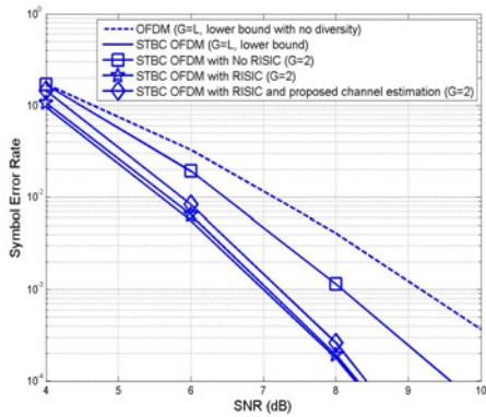
그림 8. CH_1 채널에 대한 STBC OFDM 시스템의 심볼 에러율 성능
