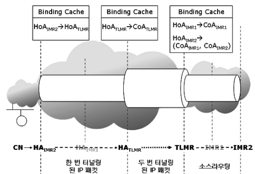
그림 2. 대응단말에서 이동 네트워크 단말로의 정방향 라우팅 경로 최적화
