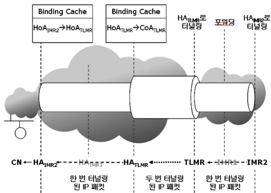
그림 3. 이동 네트워크 단말에서 대응 단말로의 역방향 라우팅 경로 최적화
