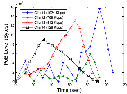
그림 5. 각 클라이언트별 재생버퍼의 상태 (기존 방식)
