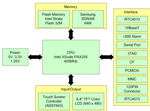
그림 9. X-Hyper255B 블록도 Fig. 9. X-Hyper255B block diagram
