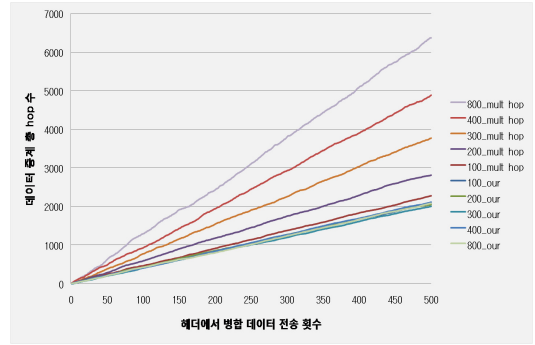
그림 4. 네트워크 노드 밀도에 따른 총 hop수의 변화
