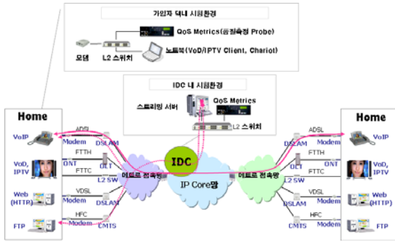
그림 1. 초고속인터넷 QoS 실증시험 환경 구성도
