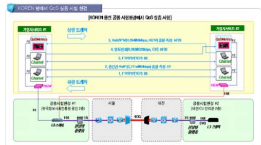
그림 7. QoS 시험환경 구성도(KOREN)
