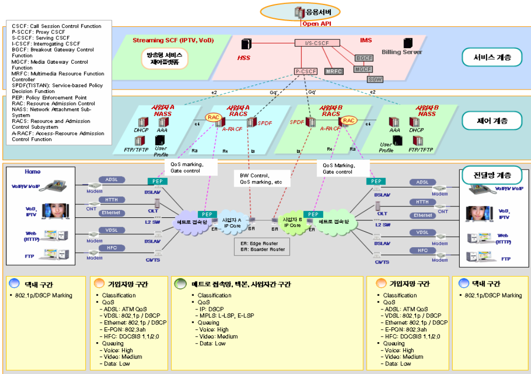
그림 6. 중단간 QoS 제공 모델
