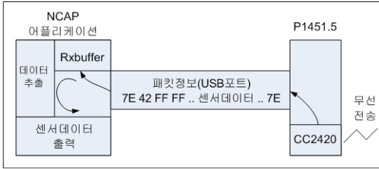
그림 6. NCAP이 센서 데이터를 읽어오는 과정
