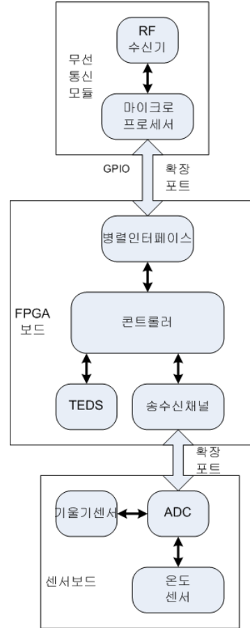
그림 7. WTIM의 블록도
