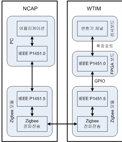
그림 2. NCAP 과 WTIM의 기능적인 구조
