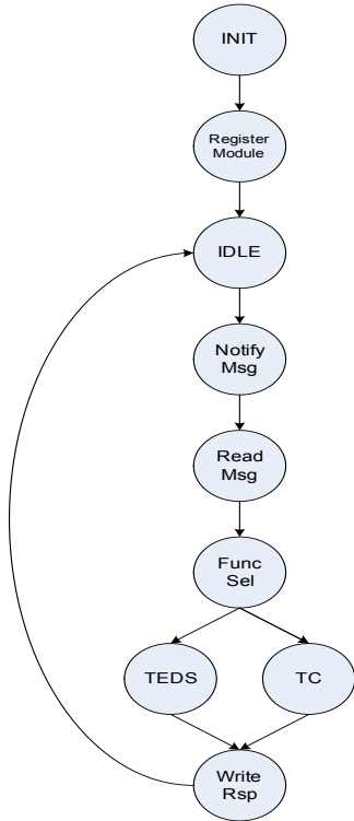
그림 8. WTIM의 상태도
