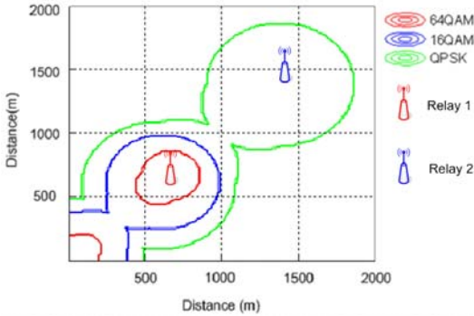
그림 11. 제안된 방식에서 단말의 수신 가능영역
