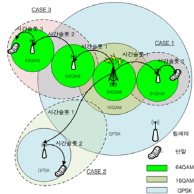
그림 2. 기존 릴레이 활용방식
