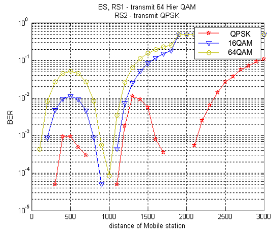
그림 8. 제한하는 방식에서 거리에 따른 단말의 수신 비트 오류율
