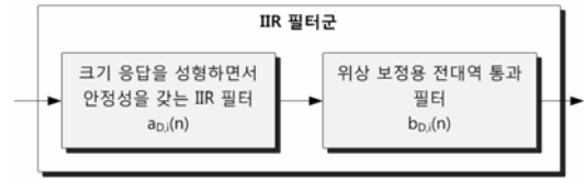
그림 3. IIR 필터군의 구조
