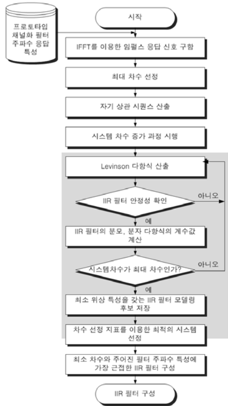
그림 4. 안정성을 보장하는 IIR 필터 설계 순서도
