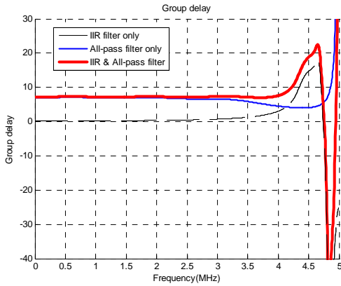
그림 8. 위상 보정용 전대역 통과 필터 유무에 따른 그룹 지연 비교
