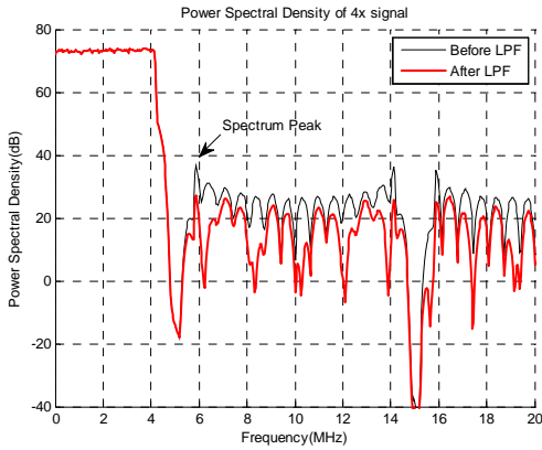
그림 10. 스펙트럼 피크 제거를 위한 저역통과필터 유무에 따른 스펙트럼 비교
