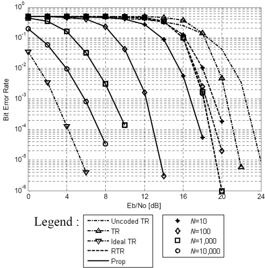
그림 5. IEEE 802.15.4a CM1에서 일반적인 TR-UWB, RTR-UWB 시스템 및 제안 기법의 BER 성능 비교 Fig. 5. Comparison of BER performances among the conventional TR-UWB, RTR-UWB systems and the proposed scheme in the IEEE 802.15.4a CM1
