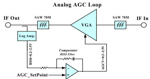
그림 2. 아날로그 AGC Loop 블록도 Fig. 2. Block Diagram of Analog AGC Loop.
