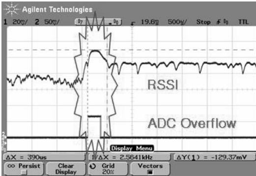
그림 10. 램프 업에서 RSSI와 ADC 오버플로 신호 Fig. 10. RSSI and ADC Overflow Flag.
