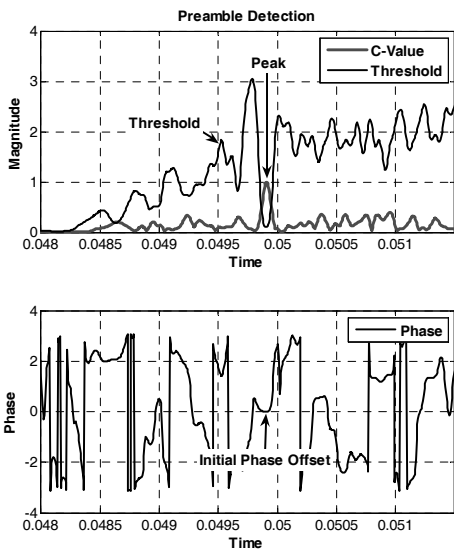
그림 21. 문턱값 및 상관기 출력 크기와 위상 Fig. 21. Threshold Value, Mag. and Phase.
