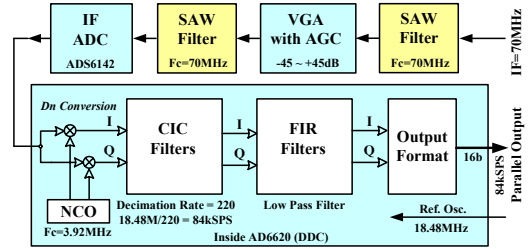
그림 1. 디지털 하향 변환기 구조 Fig. 1. Digital Down Converter.
