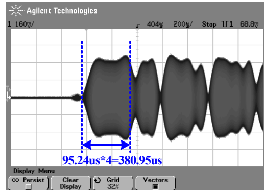
그림 5. 송신 버스트와 Ramp Up 과정 Fig. 5. Transmit Burst and Ramp Up.
