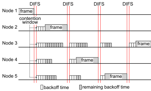
그림 3. DCF에서의 백오프 절차
