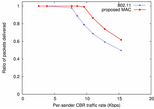
그림 9. CBR 트래픽에서 센서 노드들의 패킷 전송률
