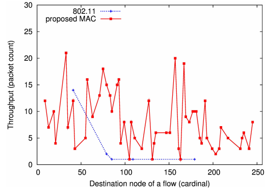
그림 8. 제안한 MAC과 802.11과의 매체 접근에 대한 공정성 비교
