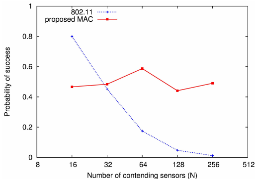
그림 7. 센서 수(N)에 따른 전송확률( p=0.6, CW=32 )
