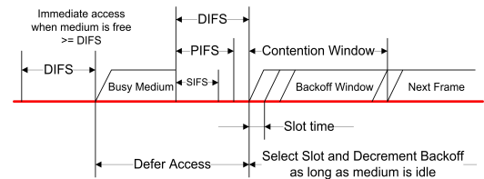
그림 2. IEEE 802.11에서 DCF를 이용한 접근 방식
