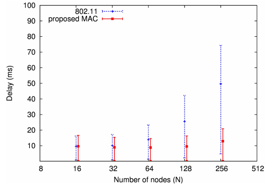
그림 10. 센서 노드의 수에 따른 전송 지연 시간의 비교
