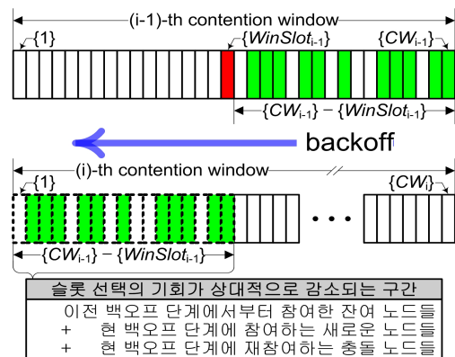
그림 4. 일반적인 BEB 방법에서의 슬롯 선택 확률 변화
