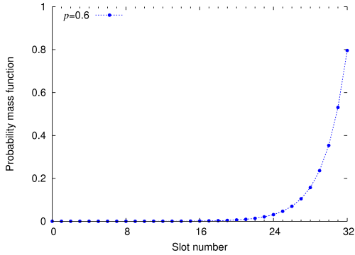
그림 6. 경쟁 윈도우 내의 슬롯 번호에 따른 확률 분포
