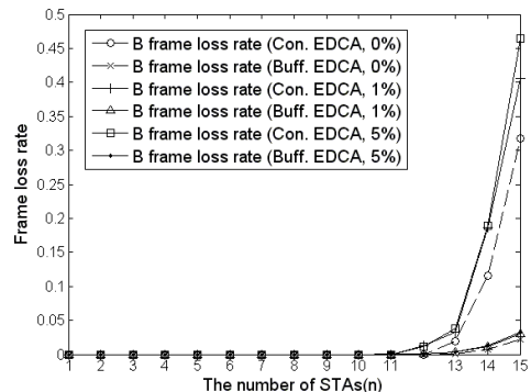
그림 13. 비디오 소스의 증가에 따른 B 프레임 손실률
