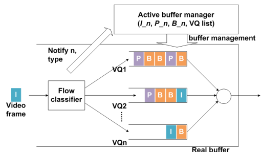
그림 6. 제안하는 동적버퍼의 구조
