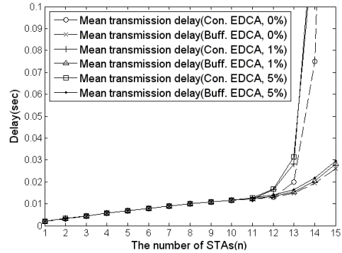
그림 10. 비디오 소스의 증가에 따른 평균 전송지연
