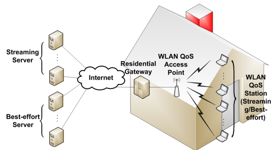
그림 4. 시스템 모델(대내 망 참조모델)
