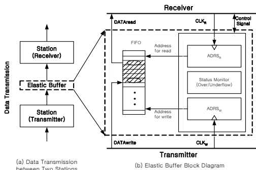
그림 1. 신축버퍼의 구성도
