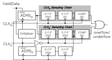
그림 2. 신축버퍼 제어부
