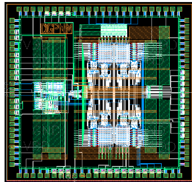
그림 5. 신축버퍼 레이아웃
