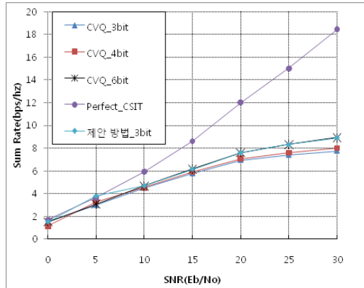
그림 5. 제안 방법과 기존 CVQ 방법의 SNR에 따른 Sum Rate 성능 그래프( M=4 )
