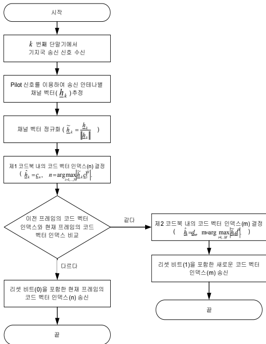
그림 3. 제안하는 피드백 방법의 순서도
