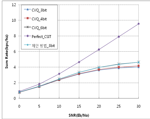
그림 4. 제안 방법과 기존 CVQ 방법의 SNR에 따른 Sum Rate 성능 그래프( M=2 )
