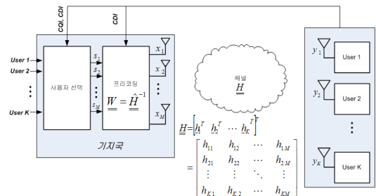
그림 1. 다중 사용자 MIMO 시스템 블록 다이어그램
