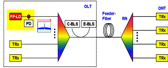
그림 4. FP-LD 모드 잠금방식(FP-LD: Fabry-Perot Laser Diode, PD:Photo-Diode, BLS: Broadband Light Source, RN: Remote Node, TRx: Transceiver)
