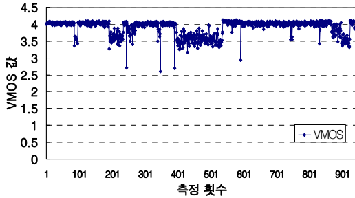
그림 10. STB에서 측정된 VMOS 측정값
