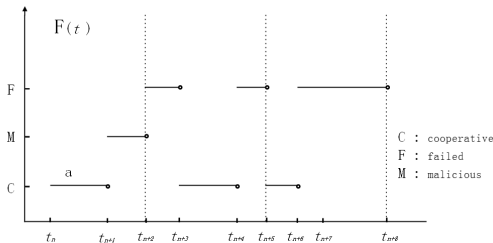
그림 1. 라우트 기능이 없는 노드의 상태 천이 견본
