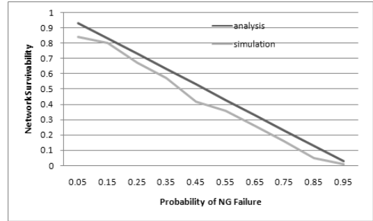
그림 9. 싱크노드의 오류가 네트워크 생존가능성에 미치는 영향
