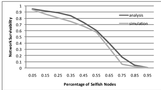
그림 7. 이기적인 노드가 네트워크 생존가능성에 미치는 영향 싱크노드로 수신되는 응용을 사용하였다.
