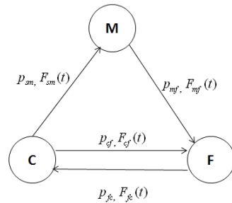
그림 4. 라우트 기능이 없는 노드에 대한 세미 마르코프 모델
