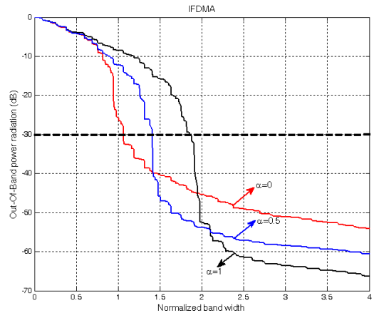
그림 4. RRC 여파기의 \alpha 에 따른 -30dB 대역폭 비교
