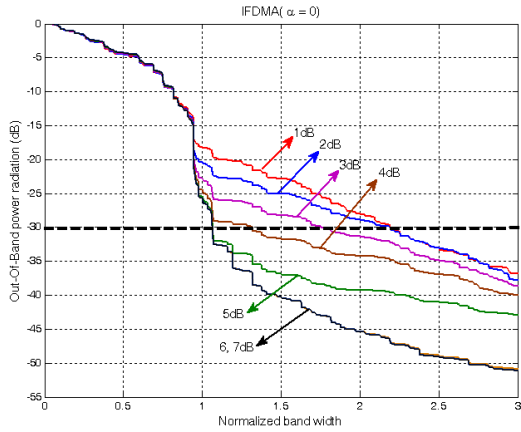
그림 5. 클리핑 임계값에 따른 스펙트럼의 변화( \alpha=0 )
