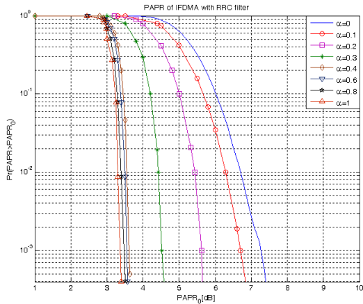
그림 3. RRC 여파기의 \alpha 에 따른 IFDMA 신호의 PAPR
