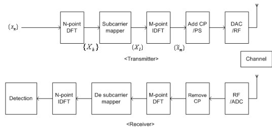
그림 1. SC-FDMA의 구조
